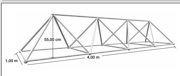
Χωροδικτύωμα
